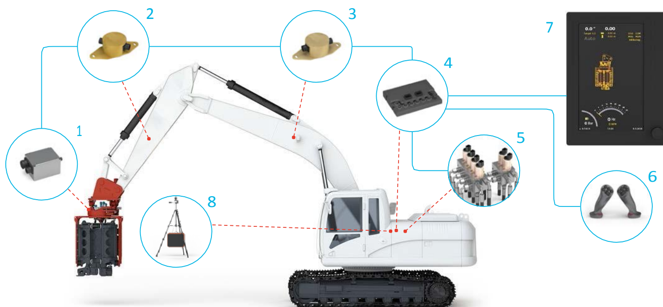
1. Модуль MOVAX
